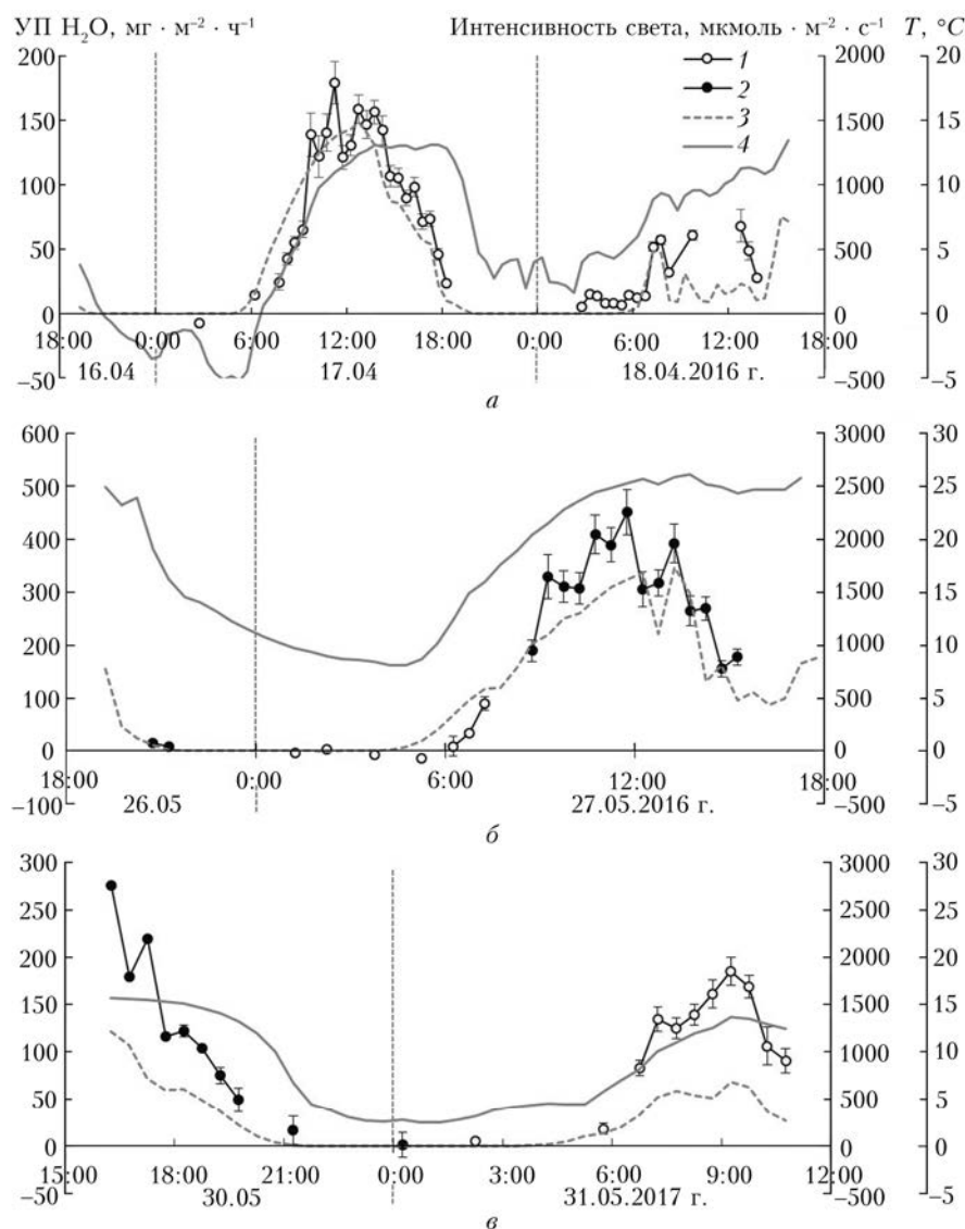
Рис. 7. УП H_2O с «южного» (1) и «северного» (2) участков; фотосинтетическая активная радиация (3); температура воздуха (4): а – апрель 2016 г.; б – май 2016 г.; в – май 2017 г.
