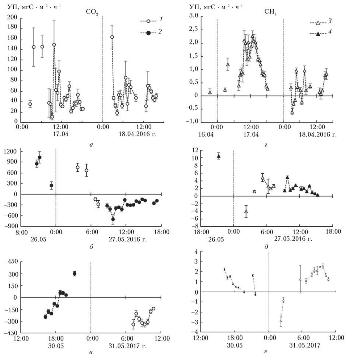
Рис. 6. УП \text{CO}_2 с «южного» (1) и «северного» (2) участков и \text{CH}_4 с «южного» (3) и «северного» (4) участков: а, з – апрель 2016 г.; б, д – май 2016 г.; в, е – май 2017 г. Значения УП отнесены к середине 30-минутного интервала усреднения; планки погрешностей соответствуют случайным погрешностям УП (см. алгоритм расчета в [32]); линии, соединяющие значения УП, даны для улучшения восприятия и не являются аппроксимацией (то же на рис. 7)
